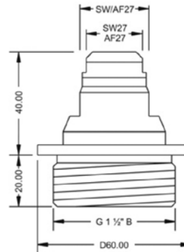
Verschlusschraube G 1 1/2“
