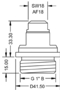
Verschlusschraube G 1“
